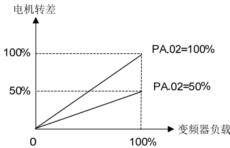
图 6-32 矢量控制 1 转差补偿增益
