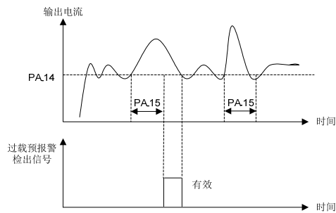
图 6-33 过载预警
