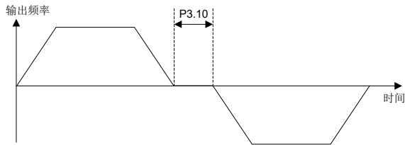
图 6-11 正反转死区时间
