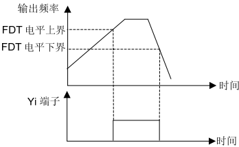
图 6-29 频率水平检测信号 FDT
