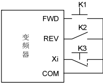
图 6-17 三线式运行模式 2
