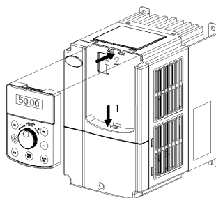
图 2-4 操作面板的安装
