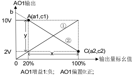
图 6-26 AO1 特性曲线 kx+b
