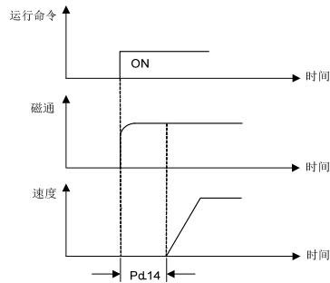
图 6-37 预激磁
