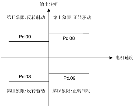
图 6-36 转矩限定
