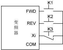
图 6-16 三线式运行模式 1
