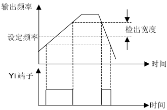
图 6-28 频率到达信号 FAR
