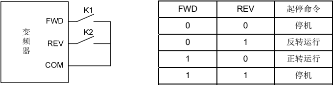
图 6-14 两线式运行模式 1
