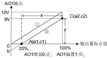
图 6-25 AO1 特性曲线 kx+b
