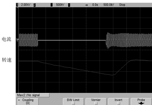
图 4 电机自由旋转时快速无冲击的转速跟踪
