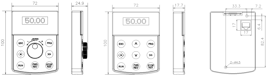
飞梭型操作面板（V6-DP01）
