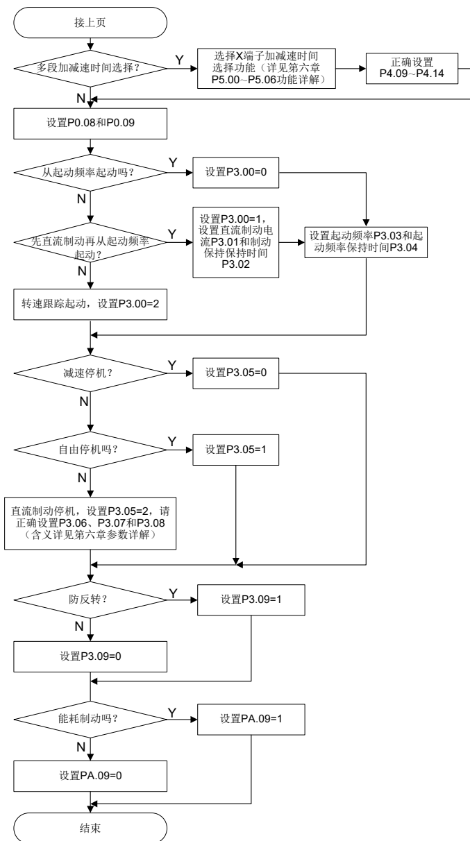
过程闭环的设置流程（续）
