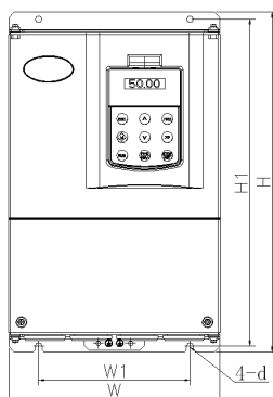
图 1-2 产品的外形和安装尺寸
