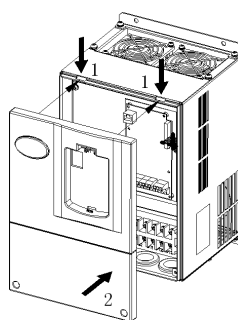
图 2-10 安装盖板
