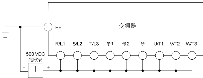
图8-2 V5-H-4T18.5 GX/22LX~V5-H-4T500GX/560LX主回路绝缘测试
