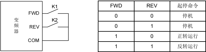
图 6-15 两线式运行模式 2
