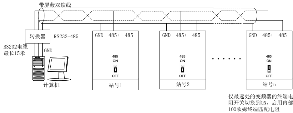
附图 4 多台变频器与计算机
