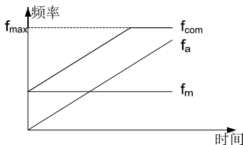
图 6-4 开环主辅给定运算 0
