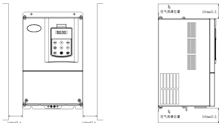
图 2-2 V5-H-4T11GX/15LX 及以上功率等级的安装方向和空间
