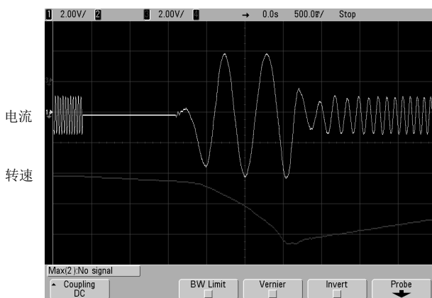
图 5 电机高速自由旋转时跟踪并降频后平滑起动
