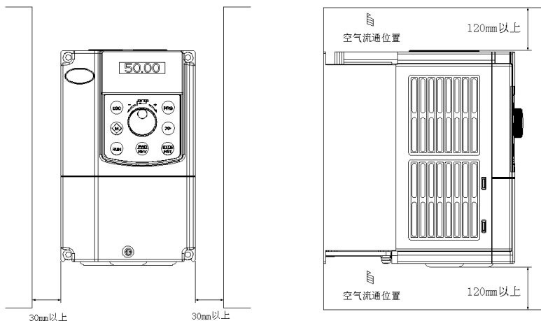
图 2-1 V5-H-2T0.4GX~V5-H-2T2.2GX 和 V5-H-4T7.5GX/11LX 及以下功率等级的安装方向和空间
