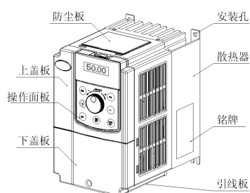
图 1-1 产品各部分的名称
