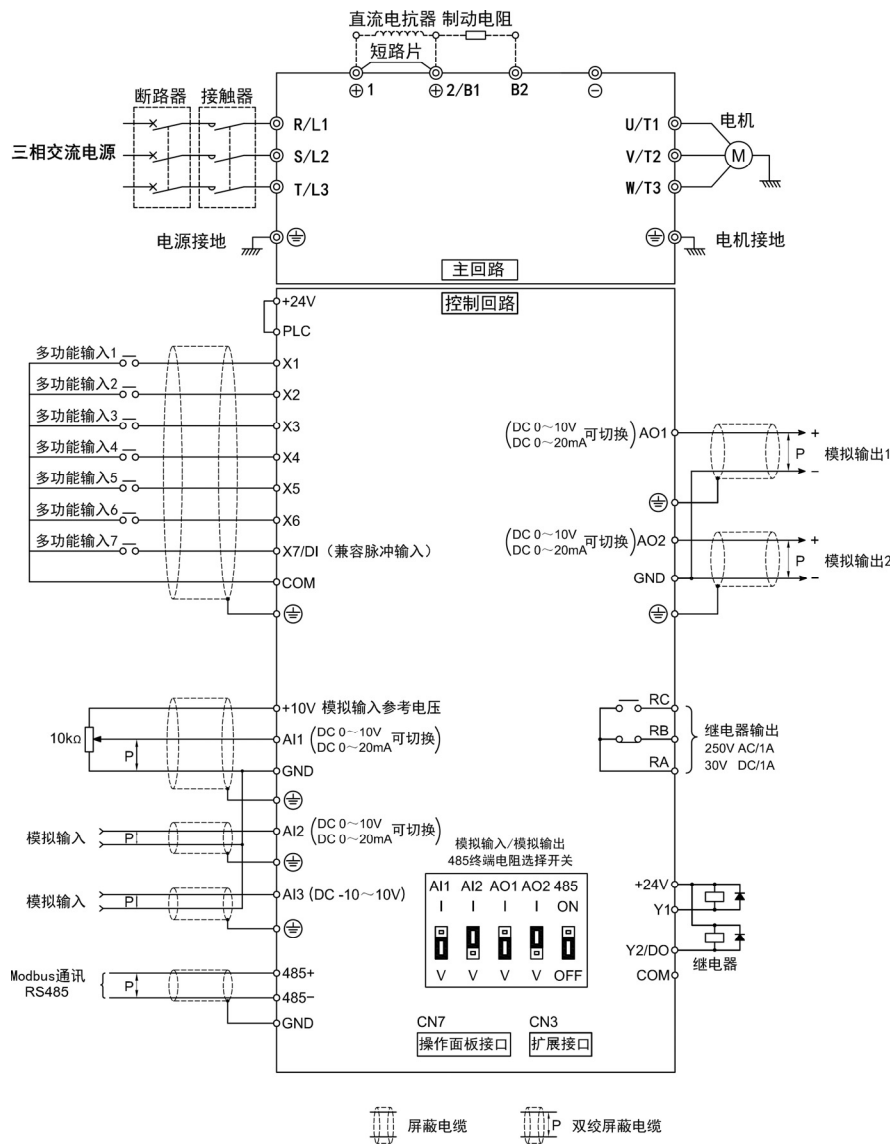
图 3-6 端子配线图 (以 V5-H-4T5.5GX/7.5LX 型举例)
