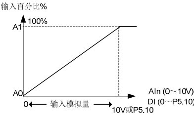
图 6-19 输入模拟量（电压/频率）对应百分比
