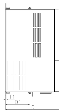
图 1-2 产品的外形和安装尺寸
