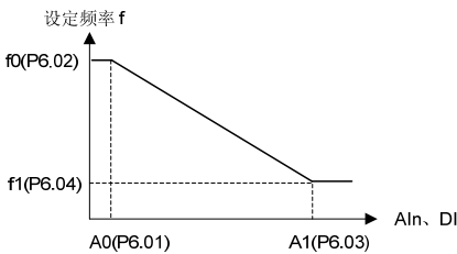
图 6-22 设定频率特性曲线（反作用）
