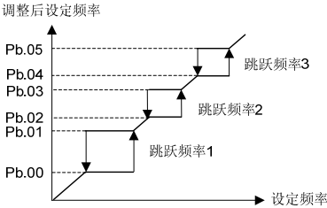
图 6-34 跳跃频率上下限
