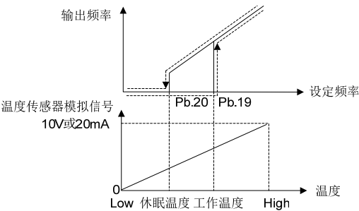
图 6-35 零频运行上下界
