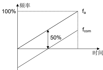
图 6-6 开环主辅给定运算 2
