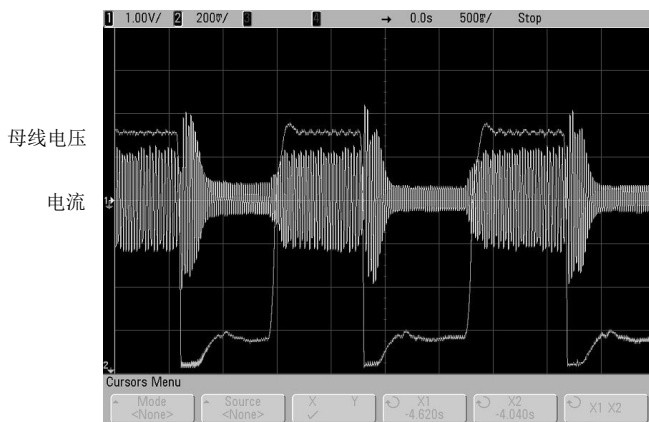
图 2 任意加减速和稳态运行，电流电压控制稳定不会跳闸保护
