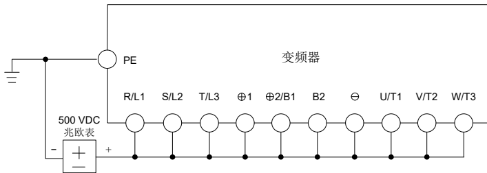
图8-1 V5-H-2T0.4GX~V5-H-2T2.2GX 、V5-H-4T0.75GX/1.5LX~V5-H-4T15GX/18.5LX 主回路绝缘测试
