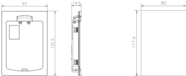
托板（V6-DP05）
