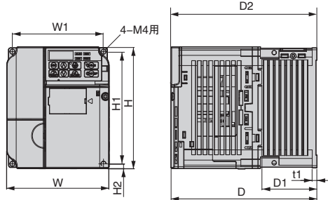
外形图2
