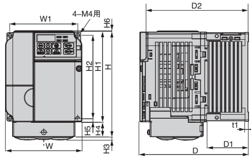
外形图 2
