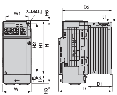
外形图 1
