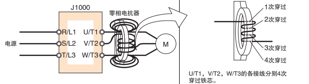
输出侧应用示例
